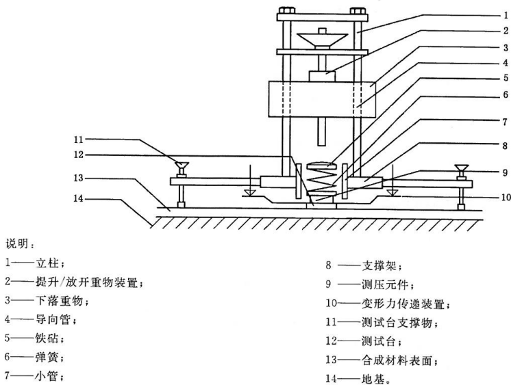
图 E.1 垂直变形测试仪
