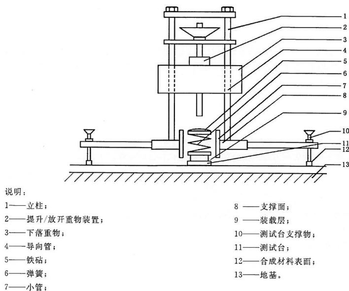
图 D.1 冲击吸收测试仪
