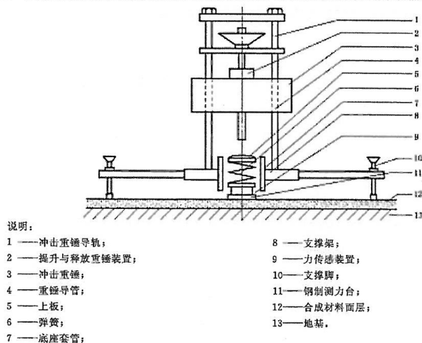
图 B.1 冲击吸收测试仪
