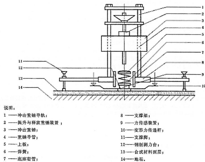
图 C.1 垂直变形测试仪
